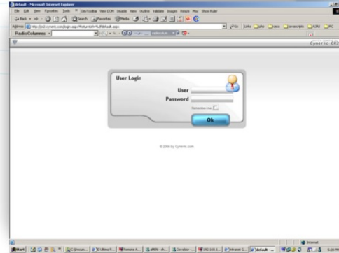
Login page
